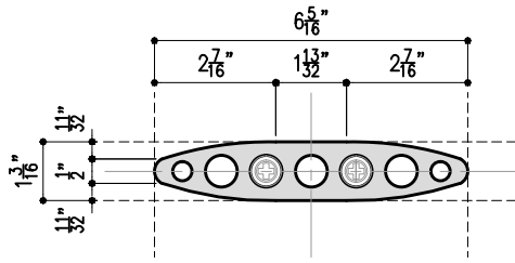
1A TC PROFILE
